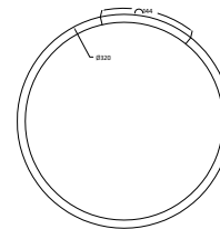
Estribo Diam.320 - Ø12
