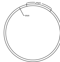
Estribo Diam.320 - Ø10
