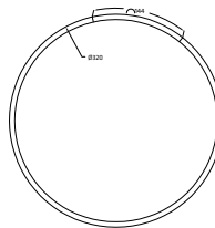
Estribo Diam.320 - Ø8
