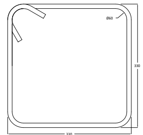
Estribo 330x330 - Ø12
