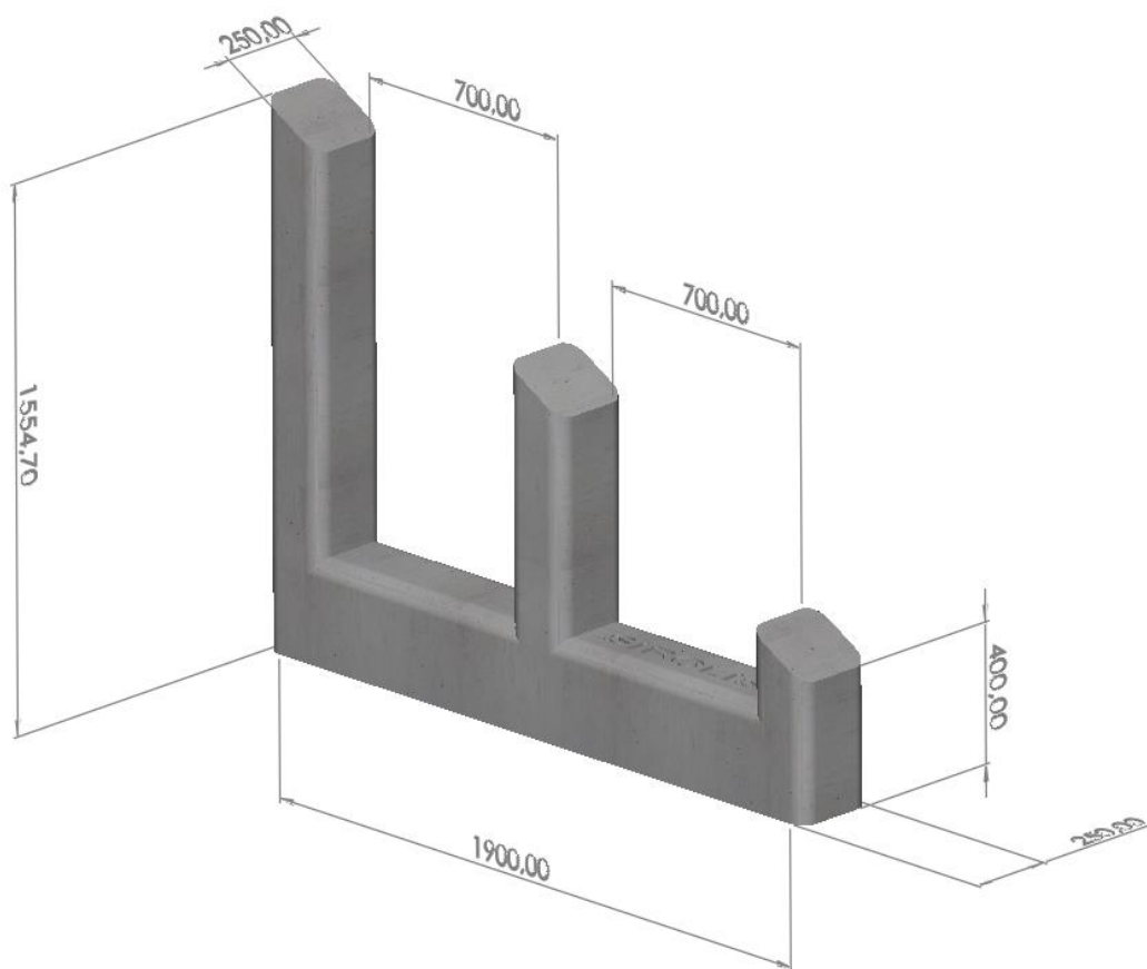
Solução com Painéis Verticais (Solution with Vertical Panels)
