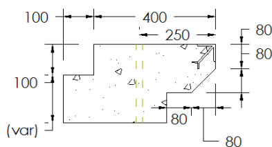
Murete Bordadura Tipo I
