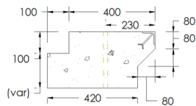
Murete Bordadura Tipo II
