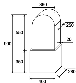
Marco Quilométrico
