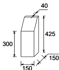
Marco Hectométrico
